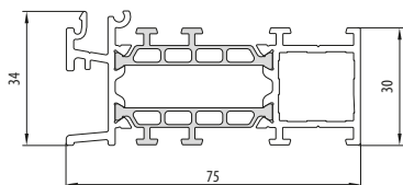
ALIPLAST GN090
