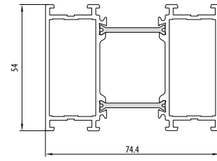
ALIPLAST SP175
