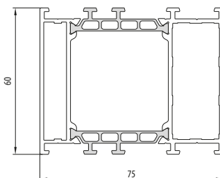
ALIPLAST GN073
